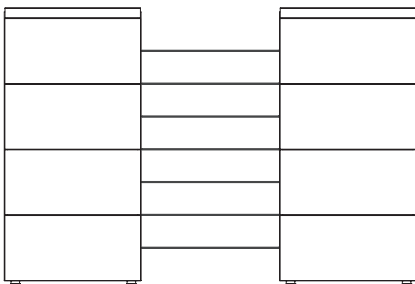
Mögliche Positionen Glasfachböden (Maße Mitte Glasboden)
